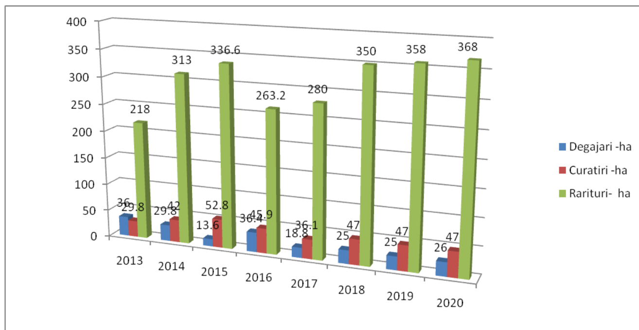
Grafic 2 – Evolutia lucrarilor de ingrijire executate anual in perioada 2013-2016 si previziuni 2017 - 2020 (hectare )
